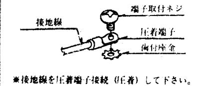
図2 接地工事
