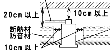
マット敷き工法
