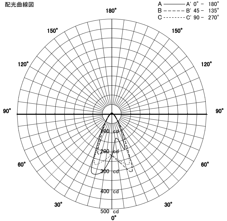
配光曲線図
