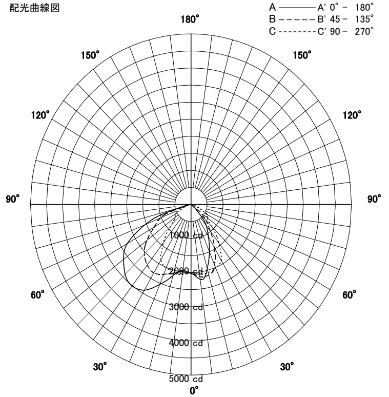
配光曲線図
