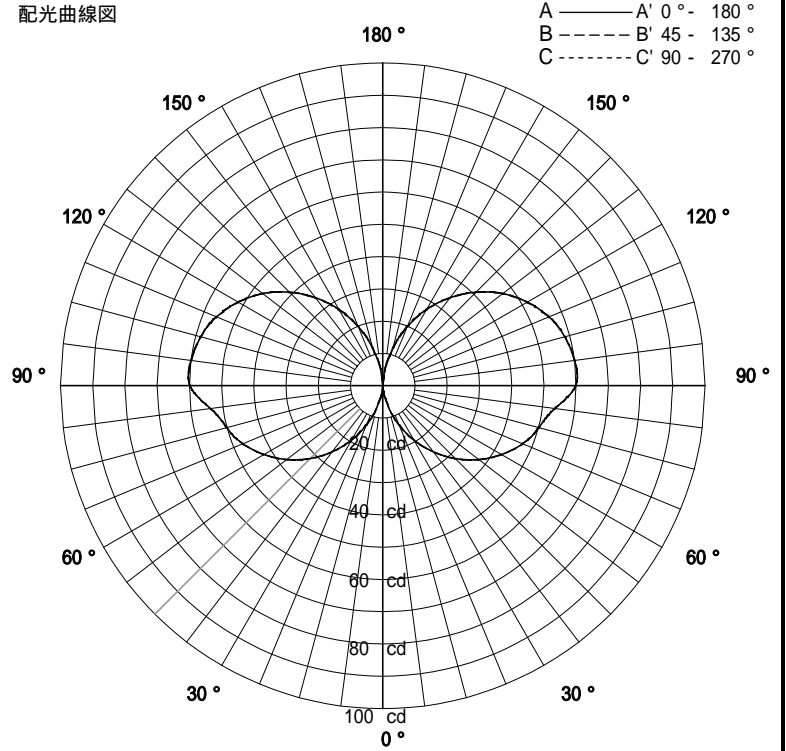
配光曲線図
