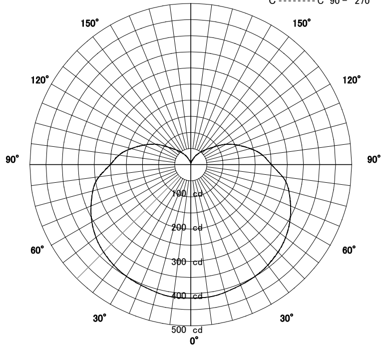
水平面照度分布
