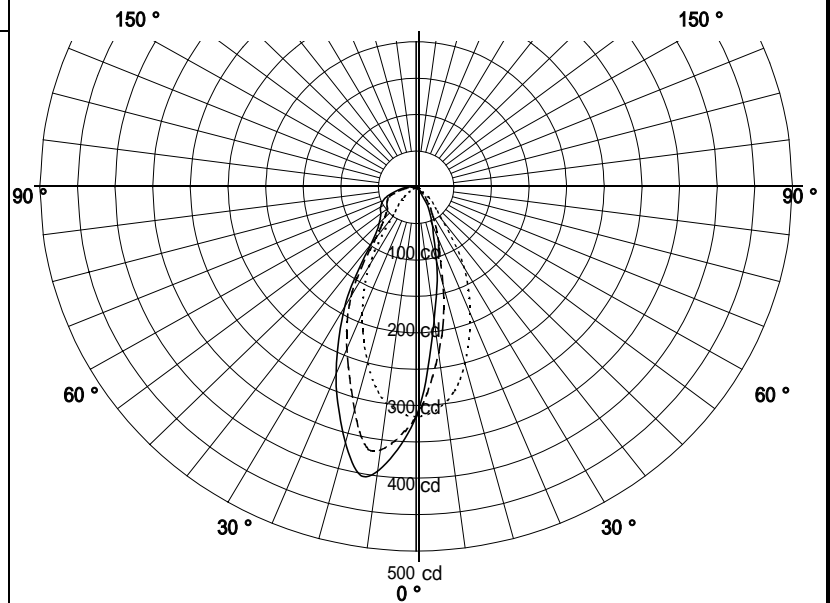
配光曲線図
