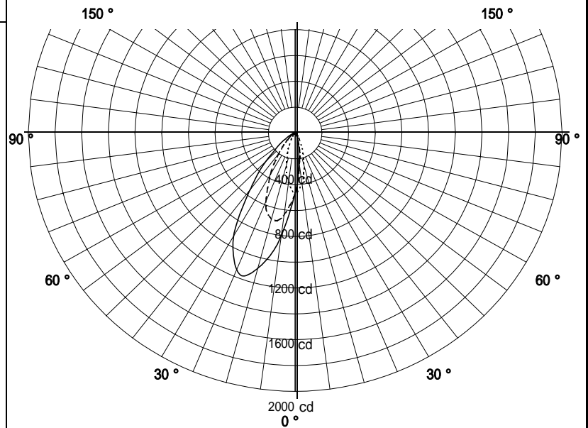
配光曲線図
