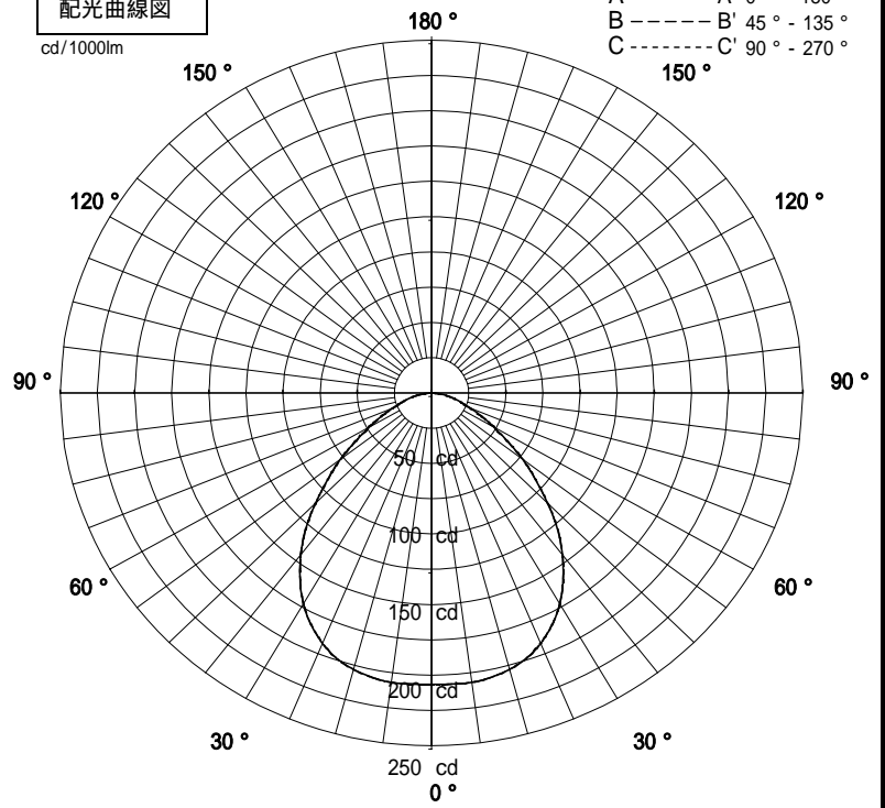
配光曲線図
