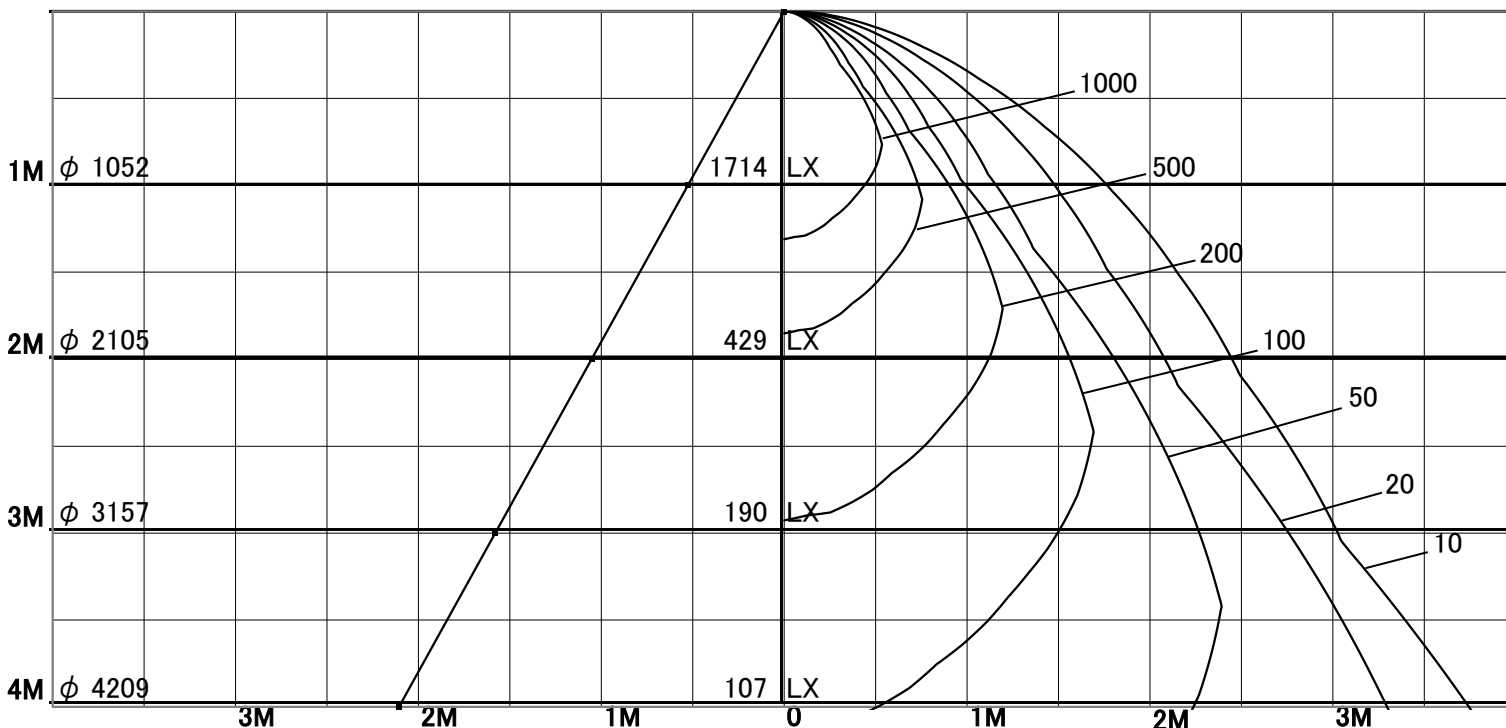
1/2照度角
