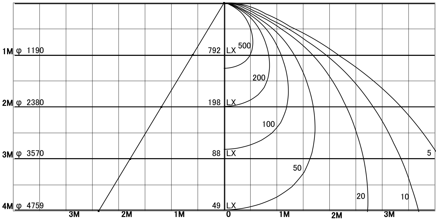
1/2照度角
