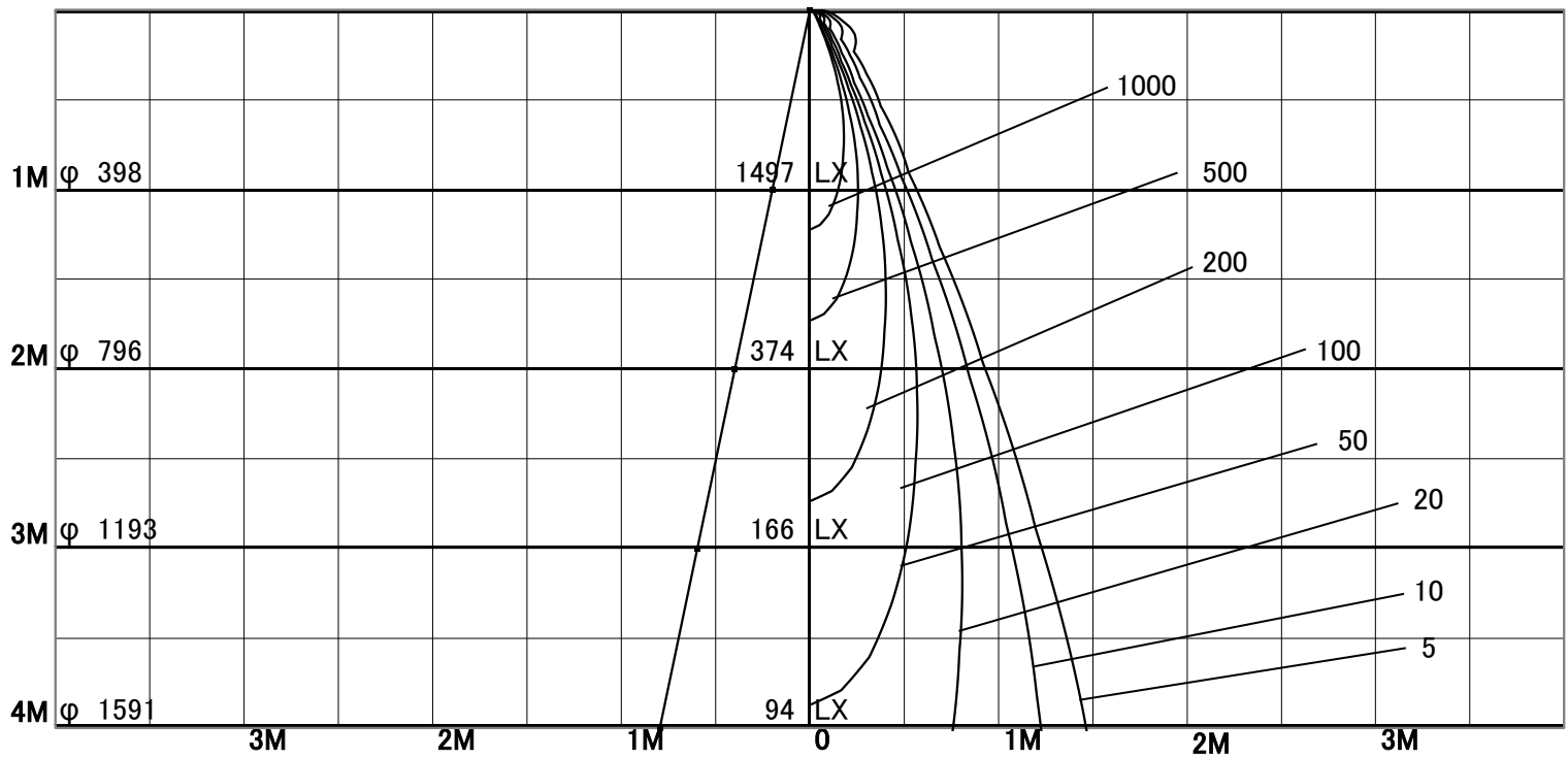
1/2照度角
