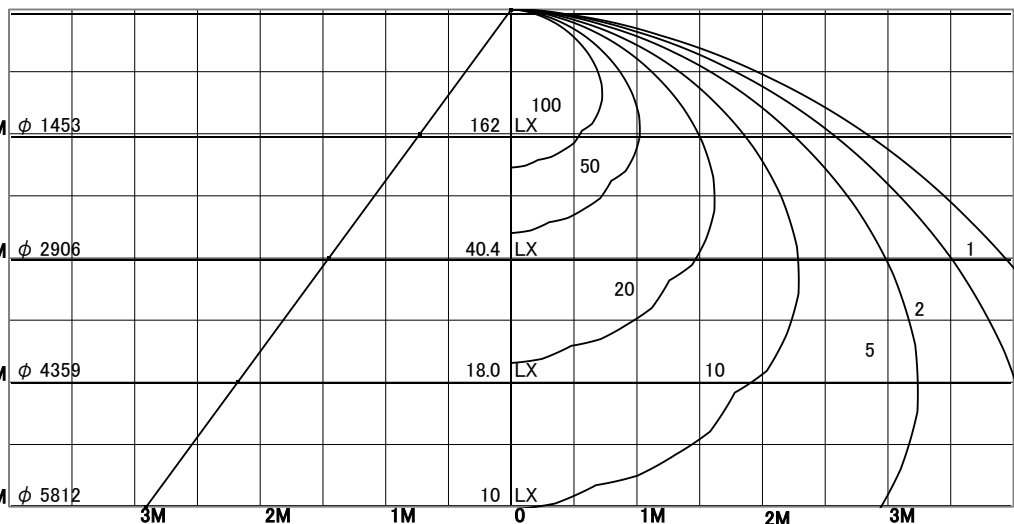
1/2照度角
