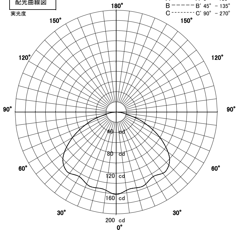
配光曲線図
