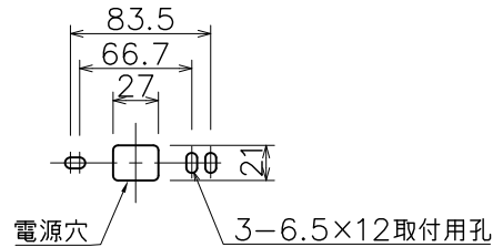
取付ピッチ(背面図)
