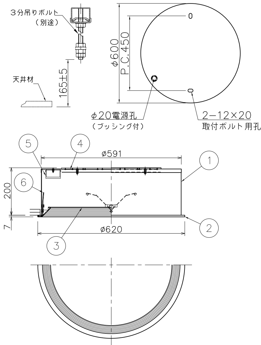
天井切込穴寸法および吊りボルトピッチ図
