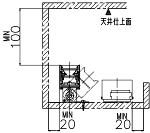
設置参考例
