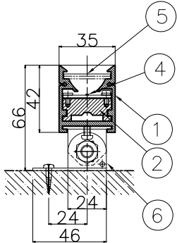
断面詳細図
