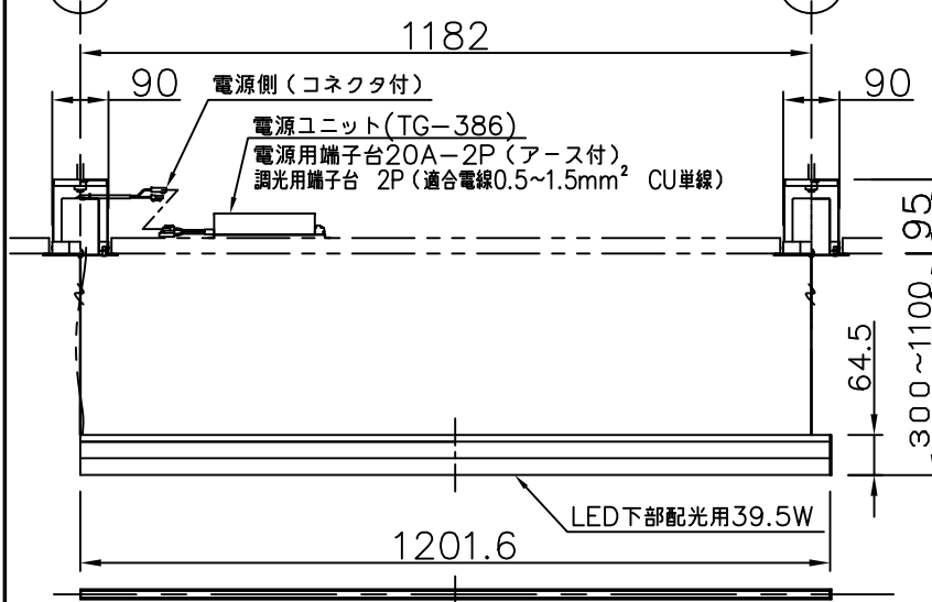
天井切込穴寸法及び取付けボルトピッチ図
