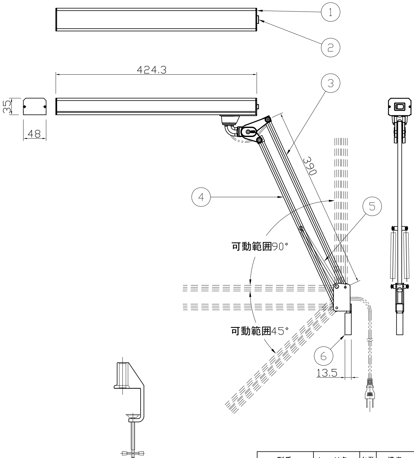
Z-A9クランプ
