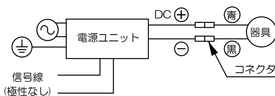
【器具接続図】
