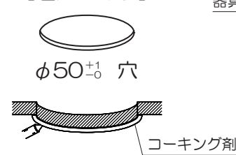
【埋込穴寸法】
