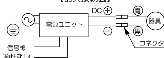
【器具接続図】
