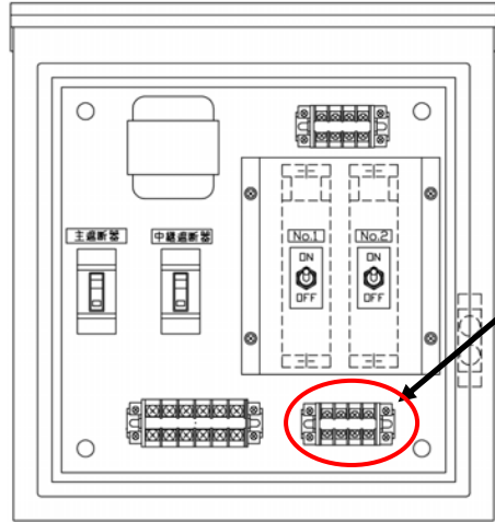
制御盤 - 内部配置図
