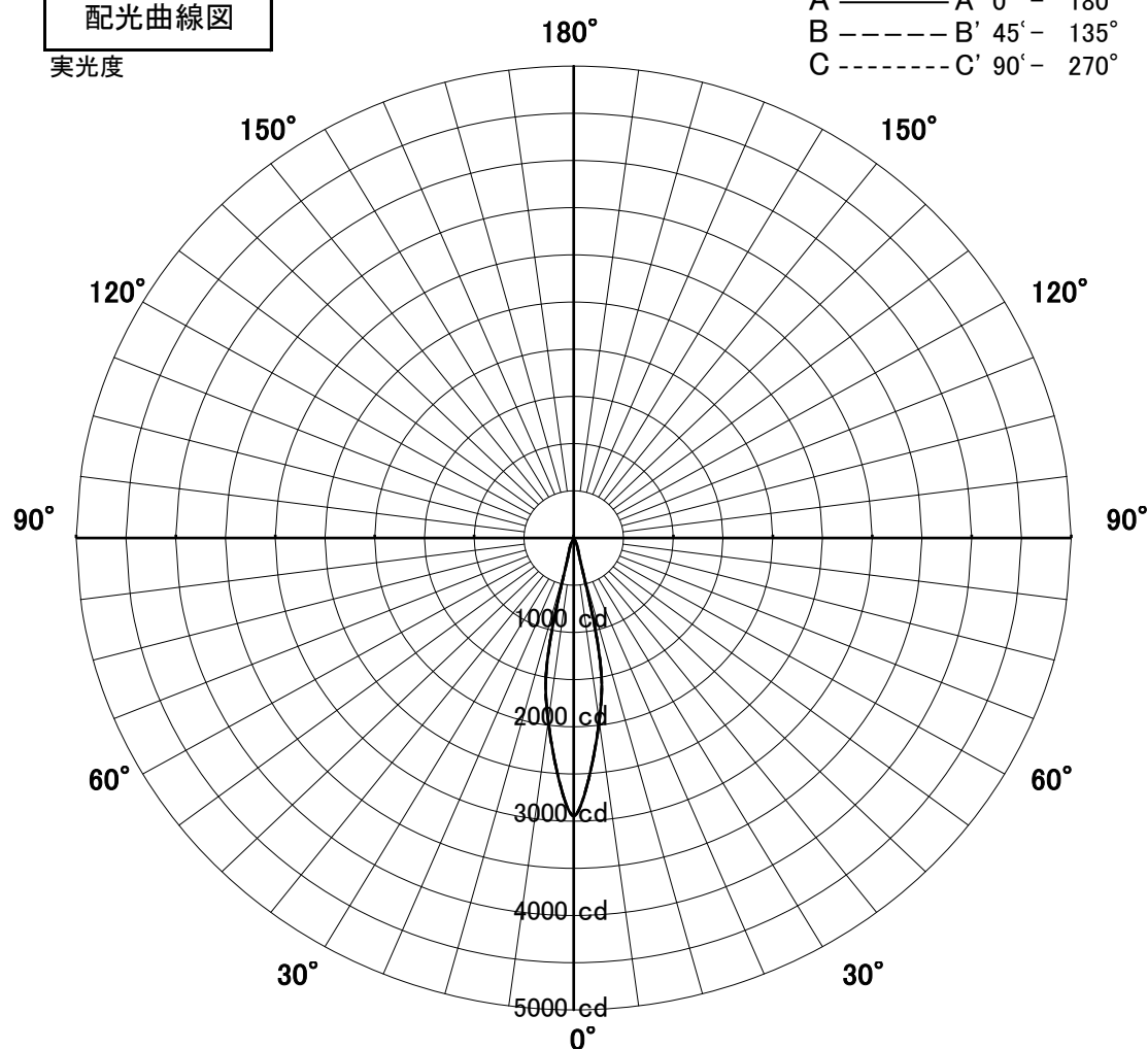
配光曲線図
