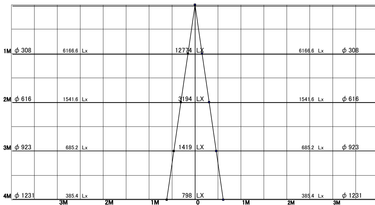
A-A' Section
