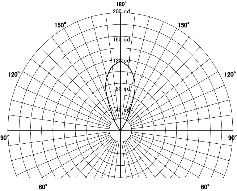
配光曲線図 実光度
