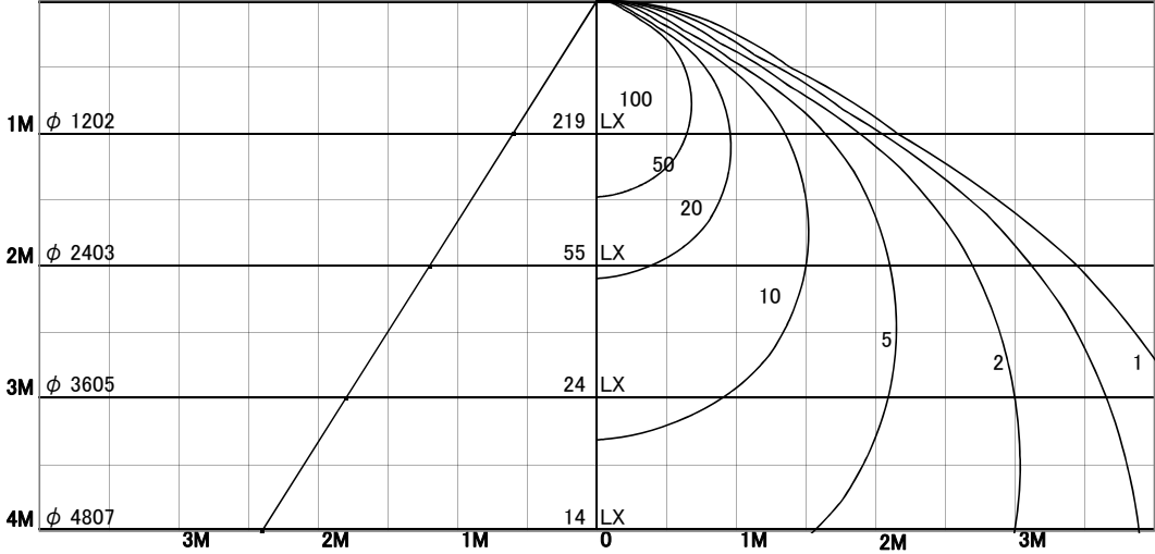
1/2照度角
