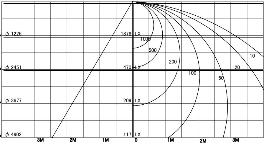
1/2照度角
