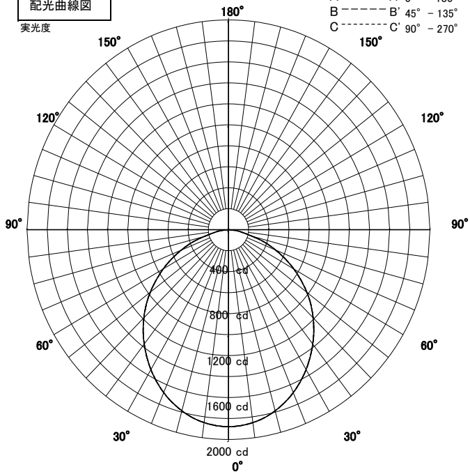
配光曲線図
