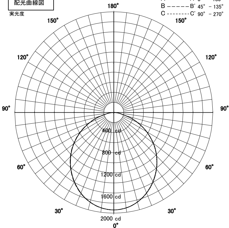
配光曲線図
