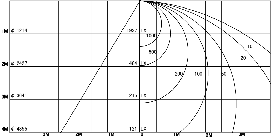
1/2照度角
