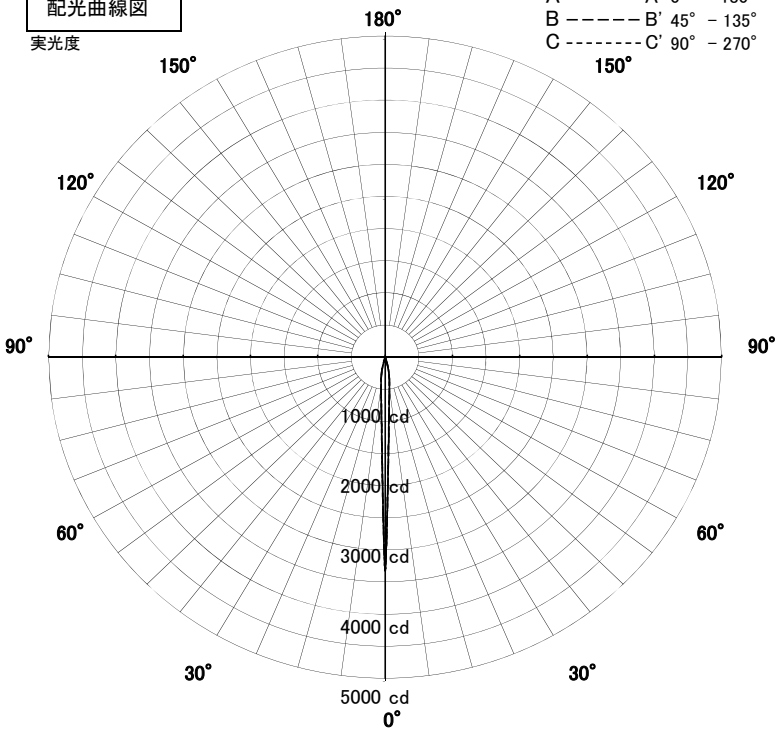
配光曲線図
