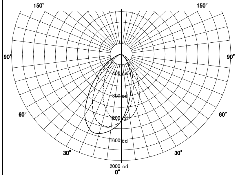
配光曲線図
