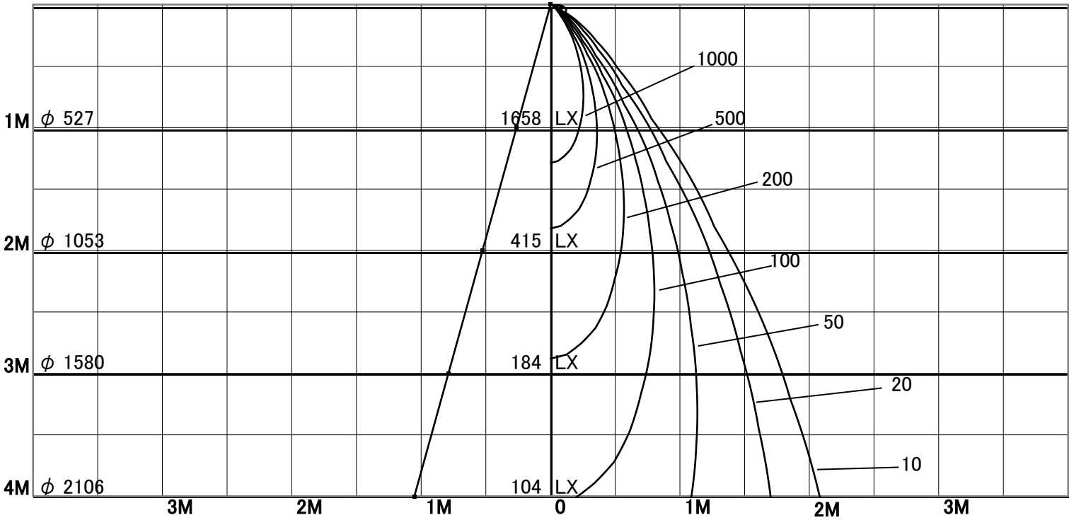
1/2照度角
