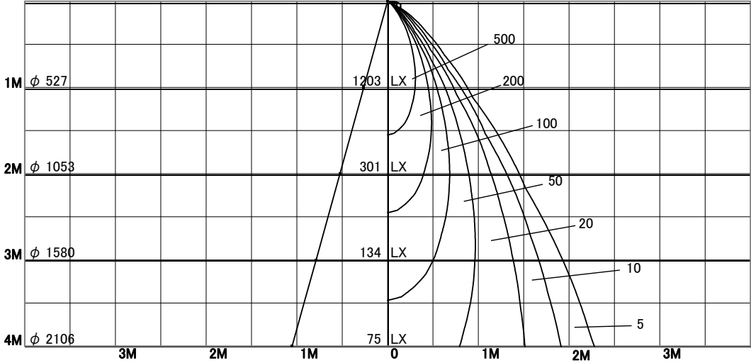
1/2照度角
