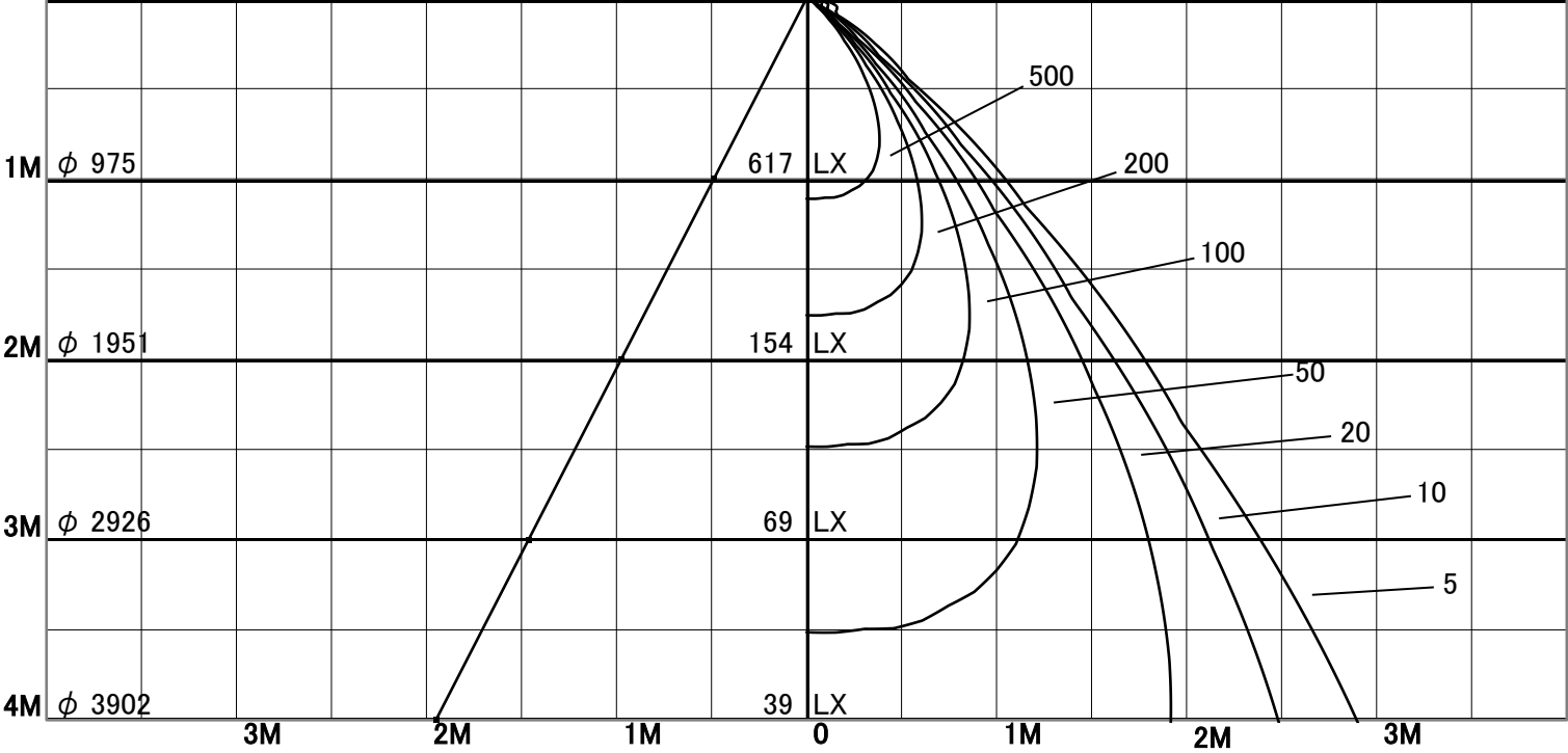
1/2照度角
