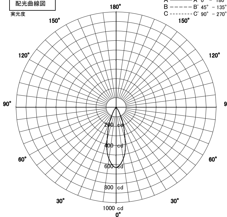
配光曲線図
