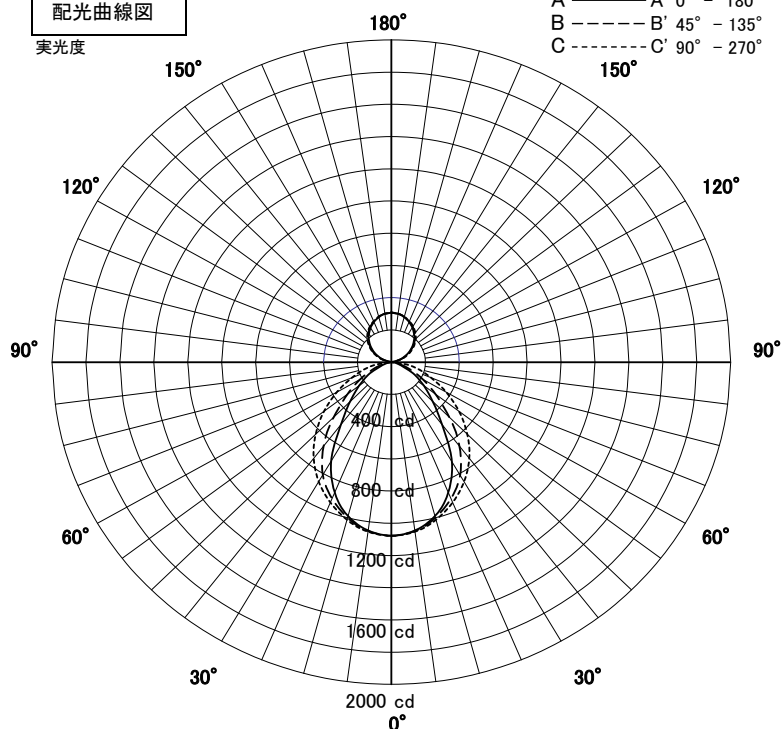
配光曲線図
