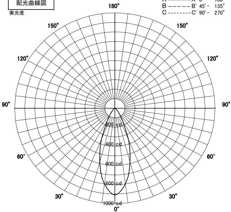
配光曲線図
