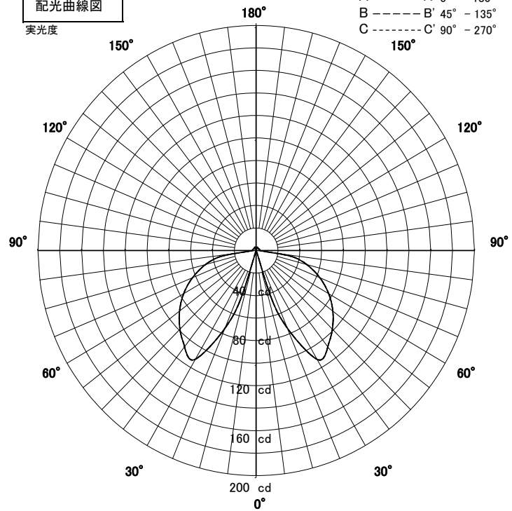
配光曲線図
