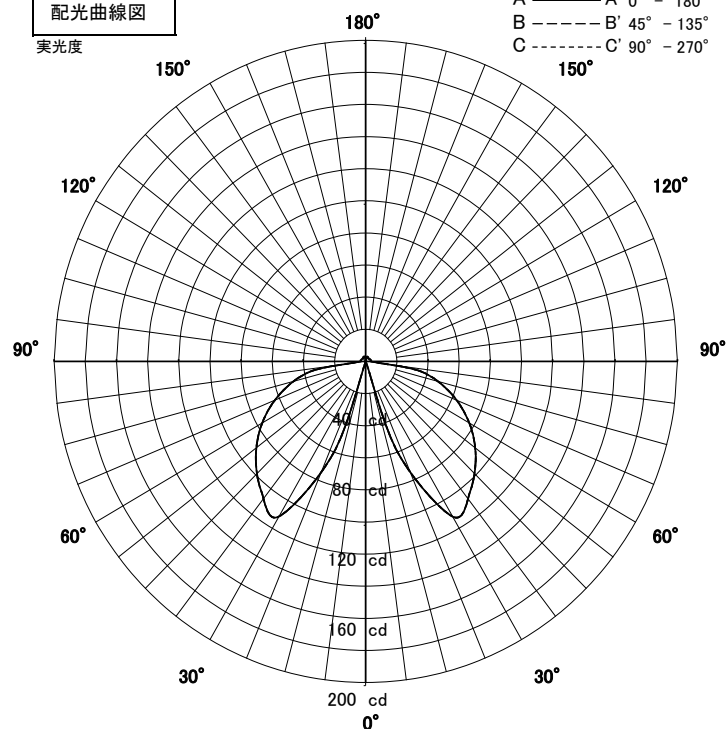
配光曲線図
