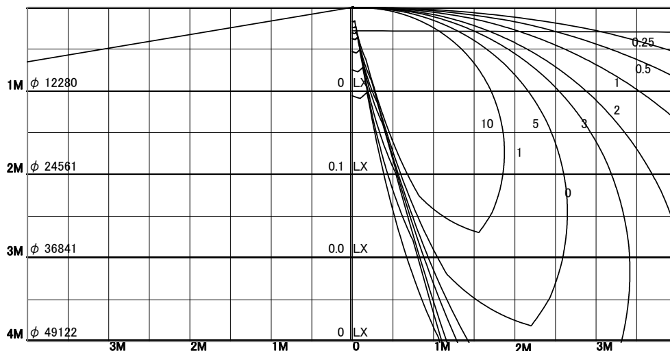
1/2照度角
