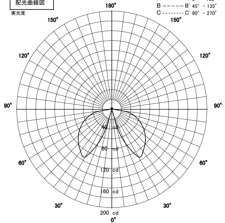
配光曲線図
