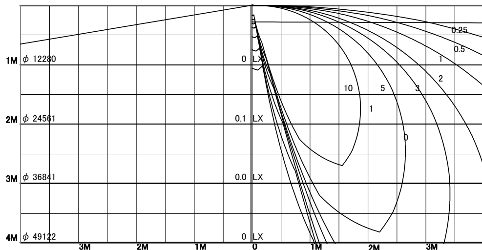
1/2照度角
